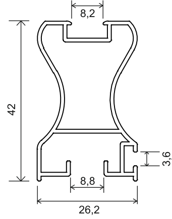
K-7565 452 gr /m
