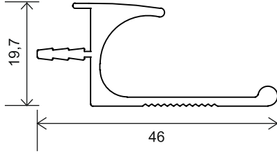
K-7510 450 gr /m
