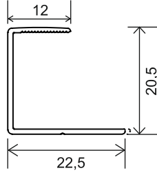
K-7570 138 gr /m
