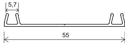
K-7545 203 gr /m
