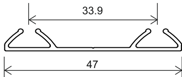
K-7540 206 gr /m
