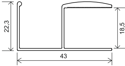
K-7575 366 gr /m
