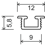
K-7585 66 gr /m
