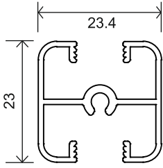
K-7530 309 gr /m
